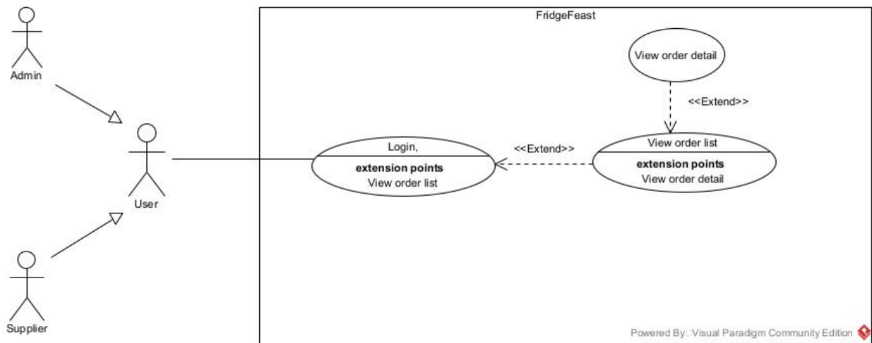
Hình 7: UC chi tiết View order list
