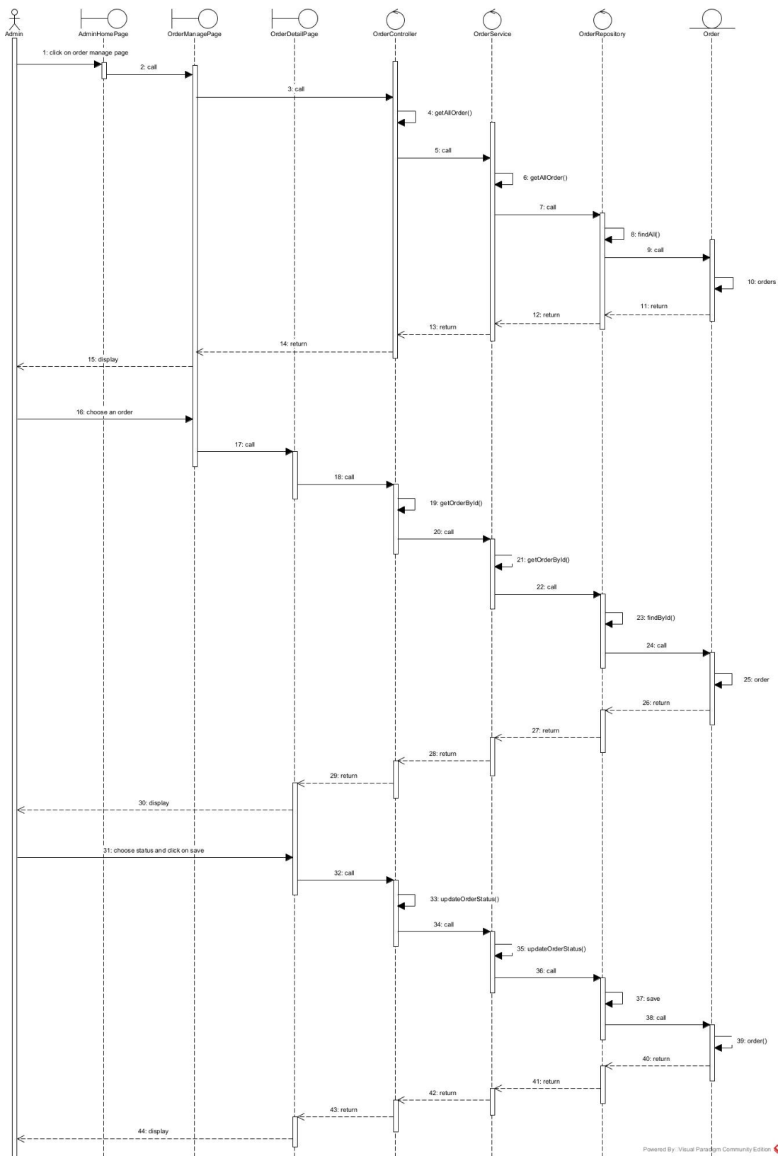
Hình 20: Sơ đồ tuần tự quản lý đơn hàng
