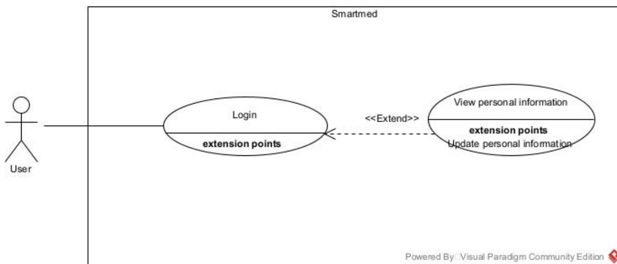
Hình 1: UC chi tiết View personal information
