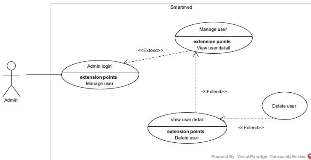
Hình 10: UC chi tiết Manage user
