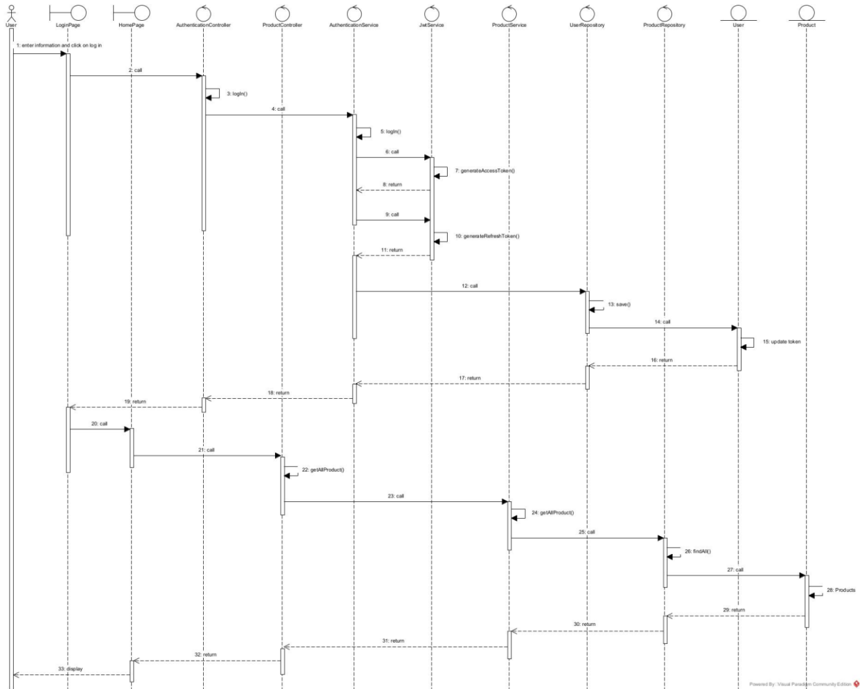
Hình 13: Sơ đồ tuần tự đăng nhập
