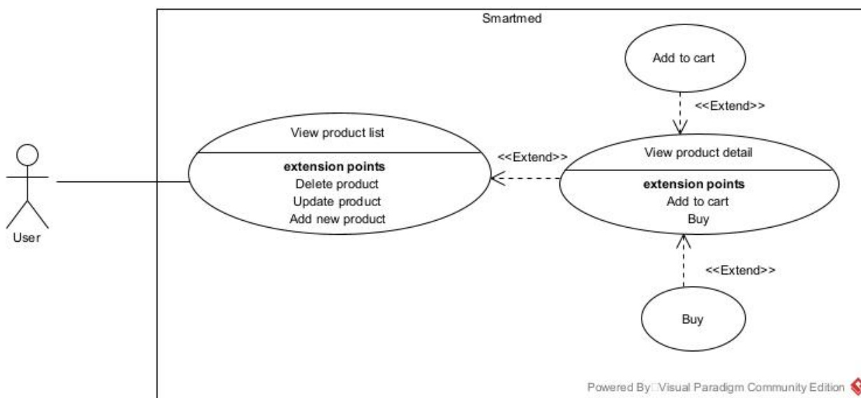
Hình 4: UC chi tiết View product detail
