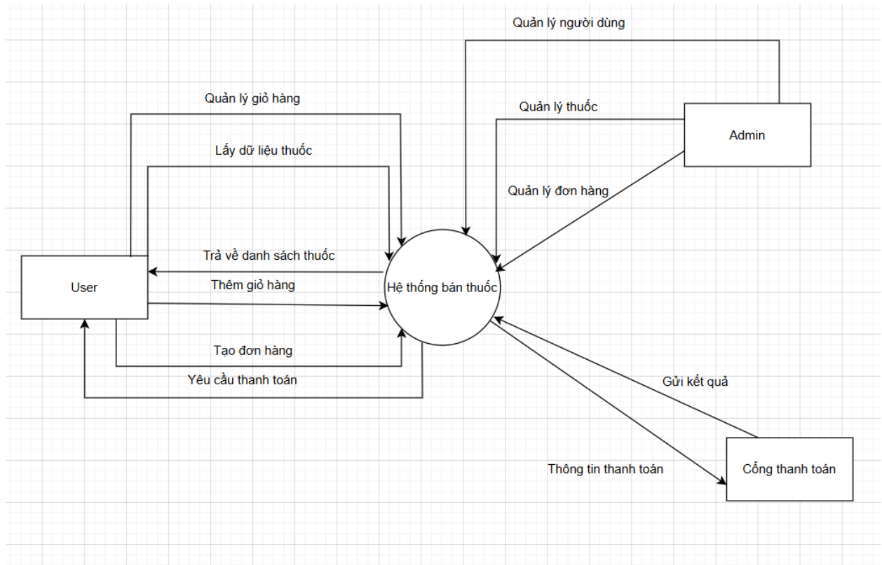
Hình 11: Sơ đồ luồng hệ thống
