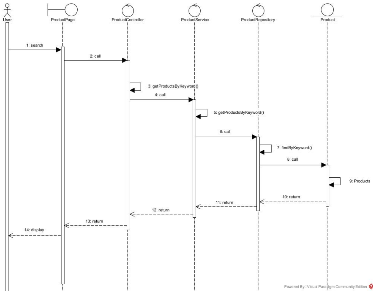
Hình 14: Sơ đồ tuần tự tìm kiếm sản phẩm
