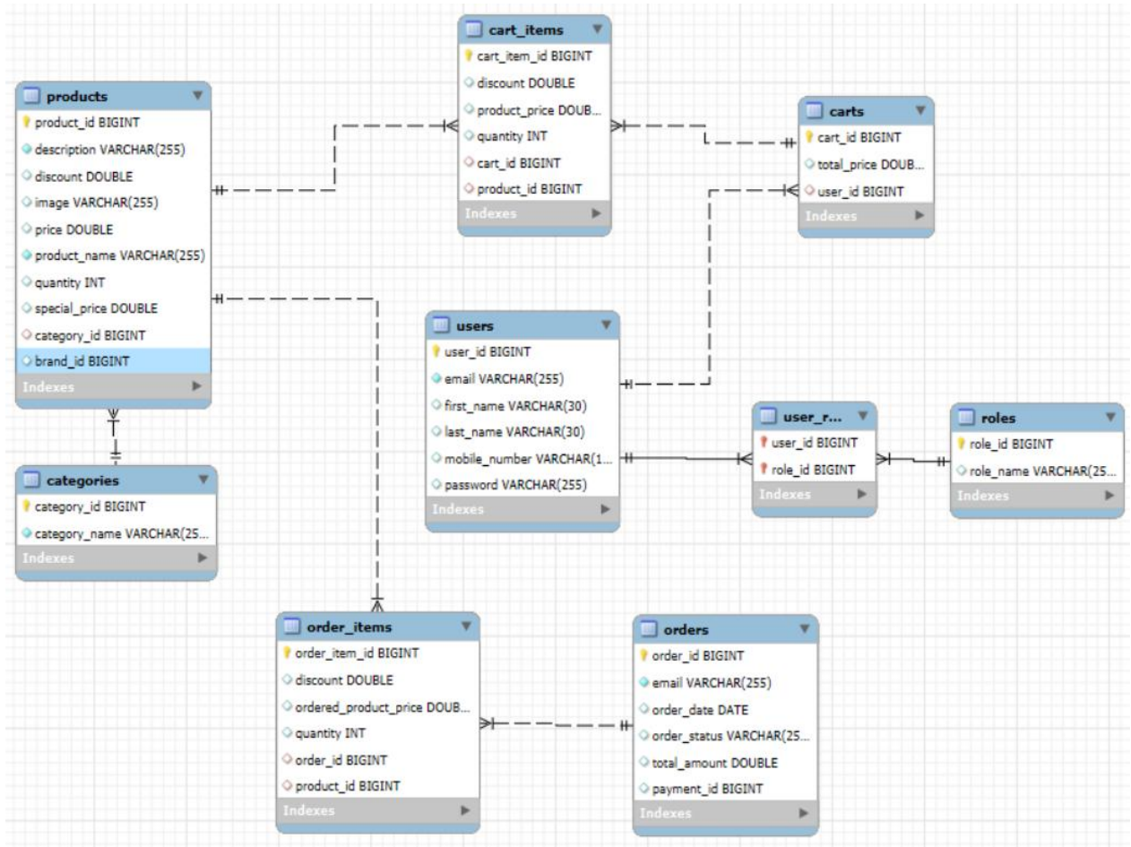
Hình 12: Cơ sở dữ liệu
